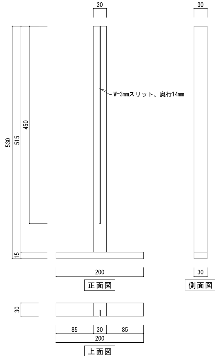
部材 B (柱部材T型) S=1/5
