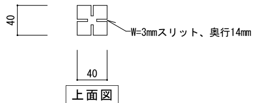
部材 A (中央部材) S=1/5
